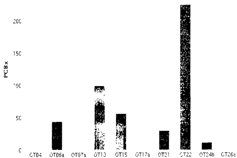
Slika 9.: Maseni udjel PCB-a u morskom sedimentu ( \mu\text{g kg}^{-1} suhe tvari) na svim postajama (Izvor: HAOP, Baza podataka i pokazatelja stanja morskog okoliša, marikulture i ribarstva)
