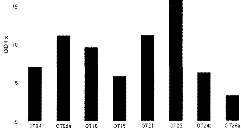
Slika 8. Maseni udjel DDT-a u morskim organizmima ( \mu\text{g kg}^{-1} suhe tvari) na svim postajama (Izvor: HAOP, Baza podataka i pokazatelja stanja morskog okoliša, marikulture i ribarstva)
