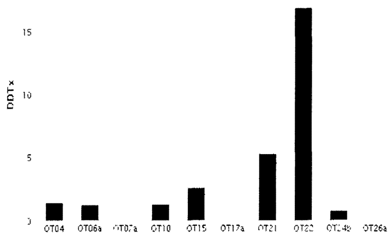
Slika 7.: Maseni udjel DDT-a u morskom sedimentu ( \mu\text{g kg}^{-1} suhe tvari) na svim postajama (Izvor: HAOP, Baza podataka i pokazatelja stanja morskog okoliša, marikulture i ribarstva)
