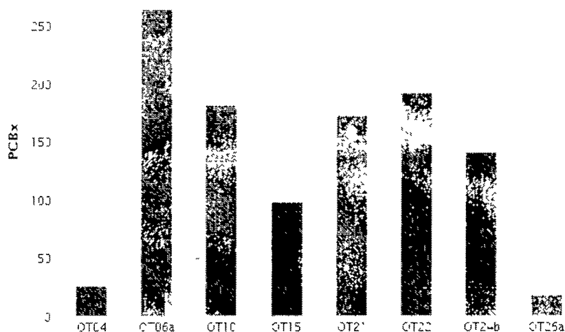
Slika 10.: Maseni udjel PCB-a u morskim organizmima ( \mu\text{g kg}^{-1} suhe tvari) na svim postajama (Izvor: HAOP, Baza podataka i pokazatelja stanja morskog okoliša, marikulture i ribarstva)
